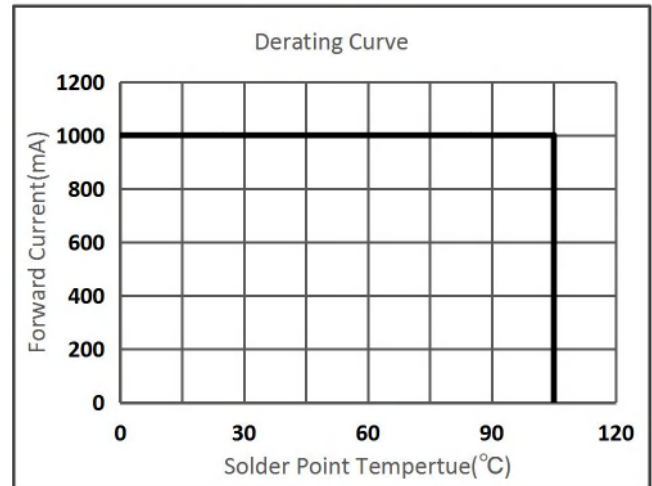
e) Derating Curve 电流下降曲线
